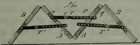
FIG 16. — Profil de la table à vivisection, dans sa deuxième position (fig. 15), pour montrer les ferrures ou tirants (T, T', T') avec leurs clous à pivot ( s ), leurs articulations ( r ) et leurs clous à tête ( p ); B, B, panneaux externes; A, A, panneaux internes (formant la gouttière).
